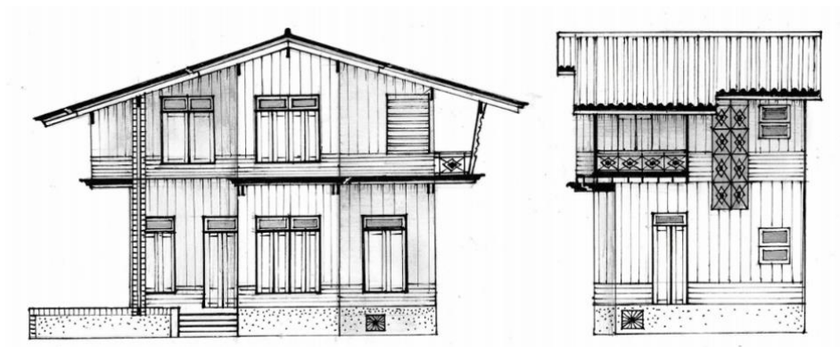
รูปที่ ๒๑๓ ลายเส้นบ้านไม้เก่า ในย่านตลาดเก่าวังทอง
