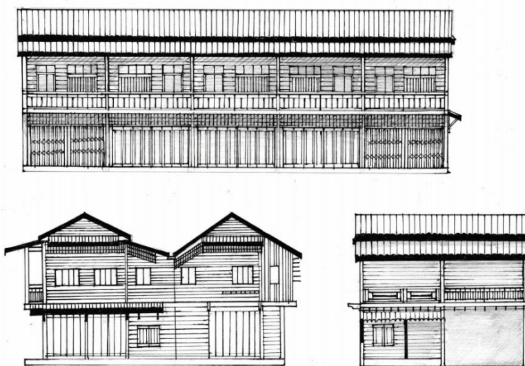
รูปที่ ๒๐๗ ลายเส้นอาคารไม้สองชั้นแบบมีระเบียง ในย่านตลาดเก่าวังทอง
